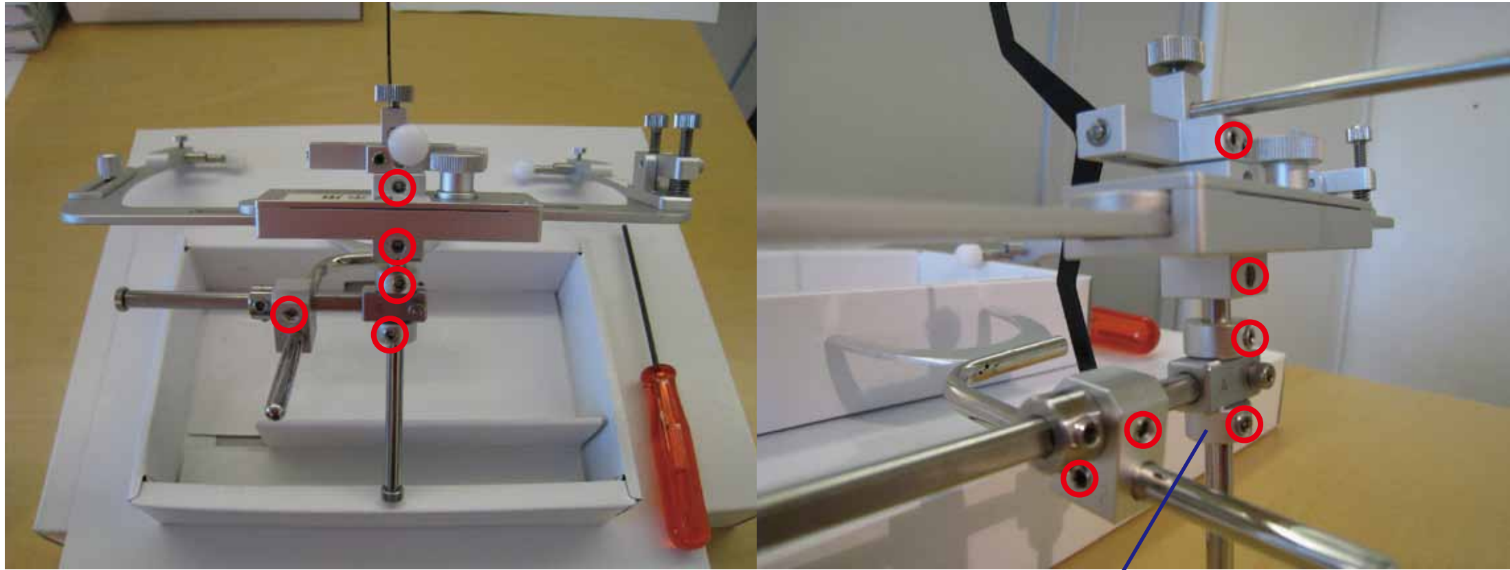
赤丸①共用六角ネジ
